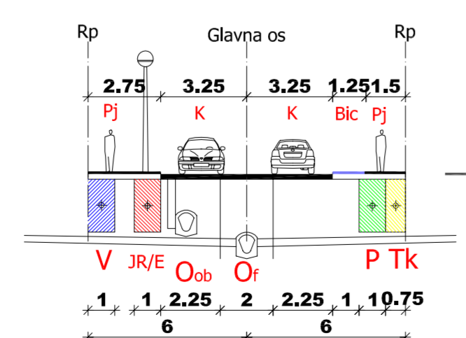
KARAKTERISTIČNI POPREČNI PRESJECI ULICA - m:1:200
